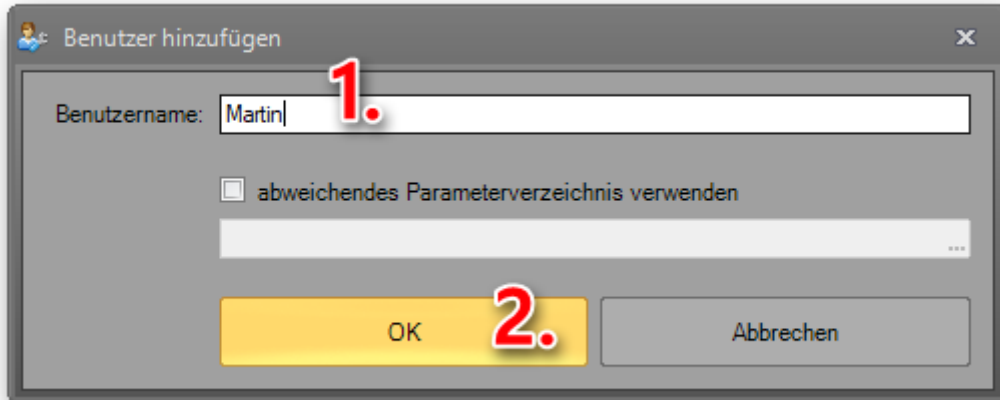
Abbildung 5: Benutzer hinzufügen
