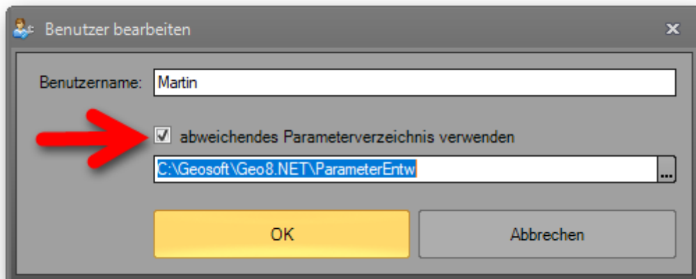
Abbildung 7: abweichender Parameterpfad
