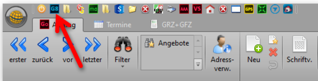
Abbildung 1: Fremdprogrammverknüpfung GEO8
