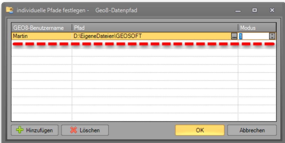
Abbildung 8: Benutzerspezifischer Speicherpfad
