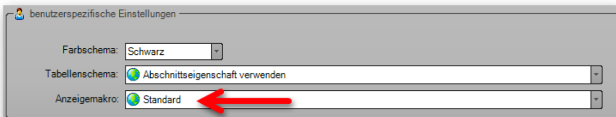
Abbildung 10: individuelles Anzeigemakro
