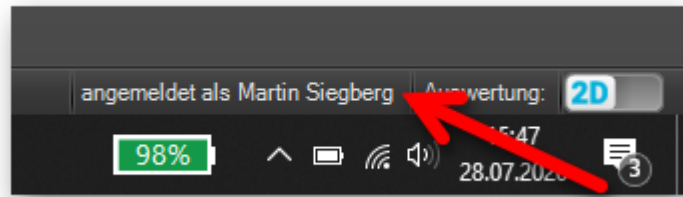
Abbildung 3: Login-Name
