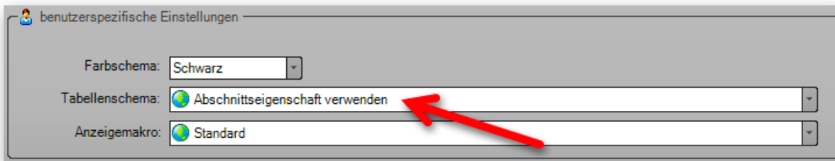
Abbildung 9: individuelles Tabellenschema
